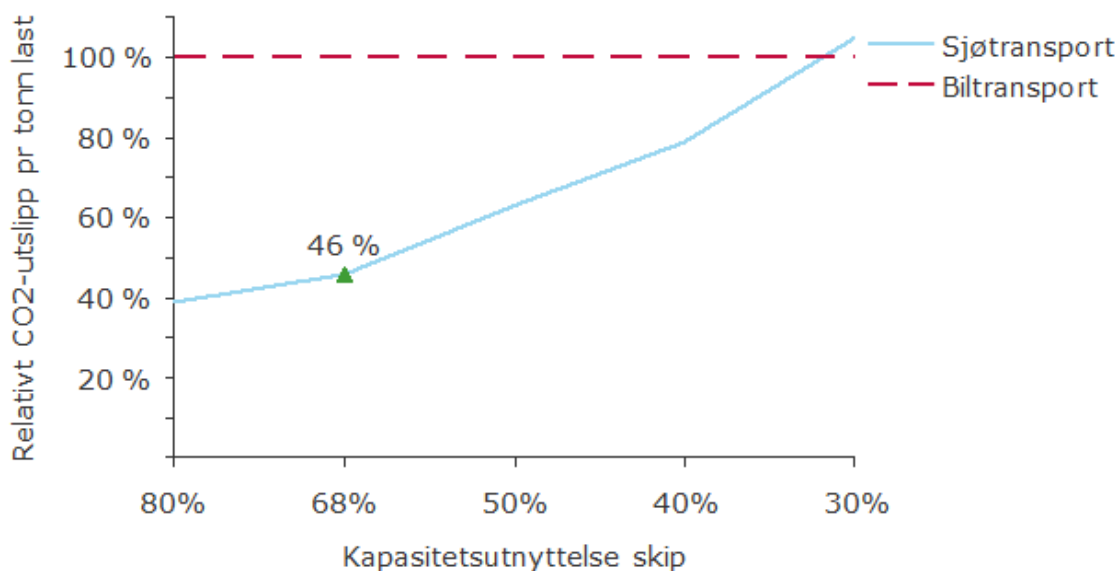
Figur 15 – Scenario 2: relativt CO 2 -utslipp med varierende kapasitetsutnyttelse for skipet
