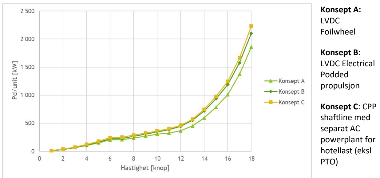
Figur 5-6: Powerkurver for tre ulike propulsjonsarrangement (tilleggsdata i vedlegg)
